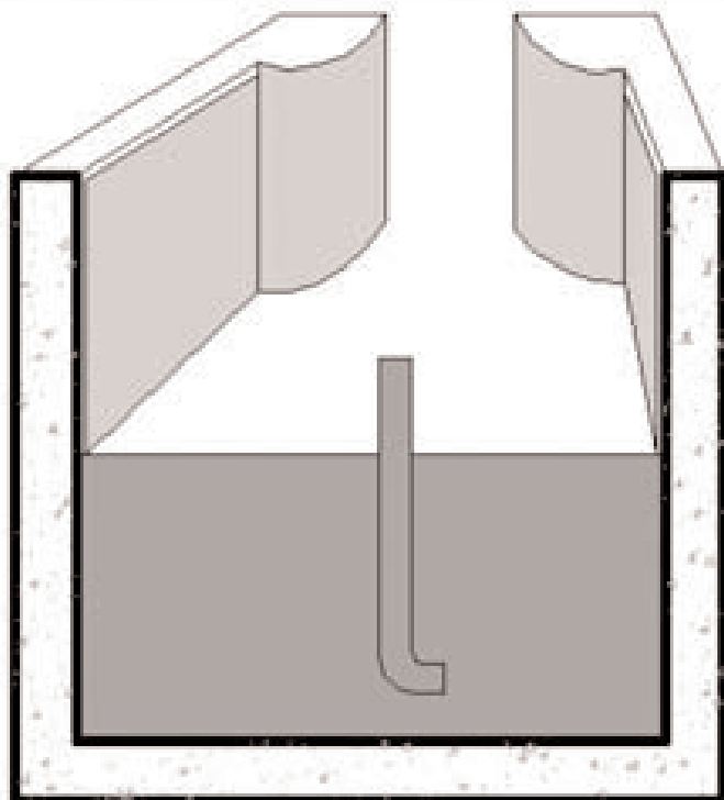
VISTA D'UNA SECCIÓ DE L'ARQUETA A
